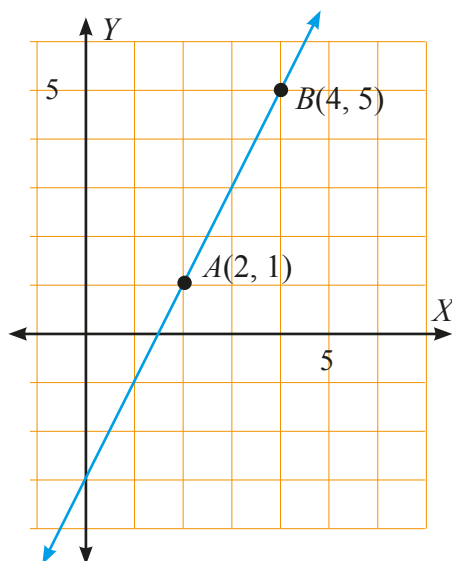
Gambar 4. 11 Garis yang kemiringannya bernilai positif
