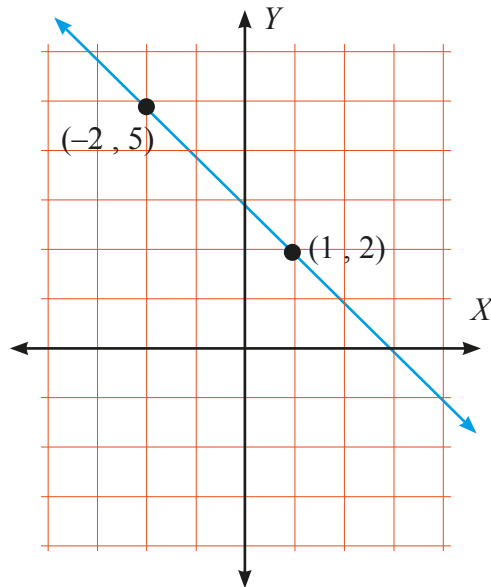
Gambar 4. 12 Garis yang kemiringannya bernilai negatif
