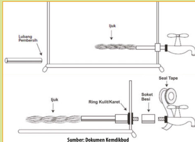
Gambar 2.19 Pipa penyaring
